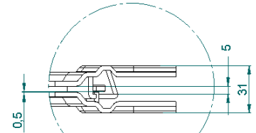
DETTAGLIO C
